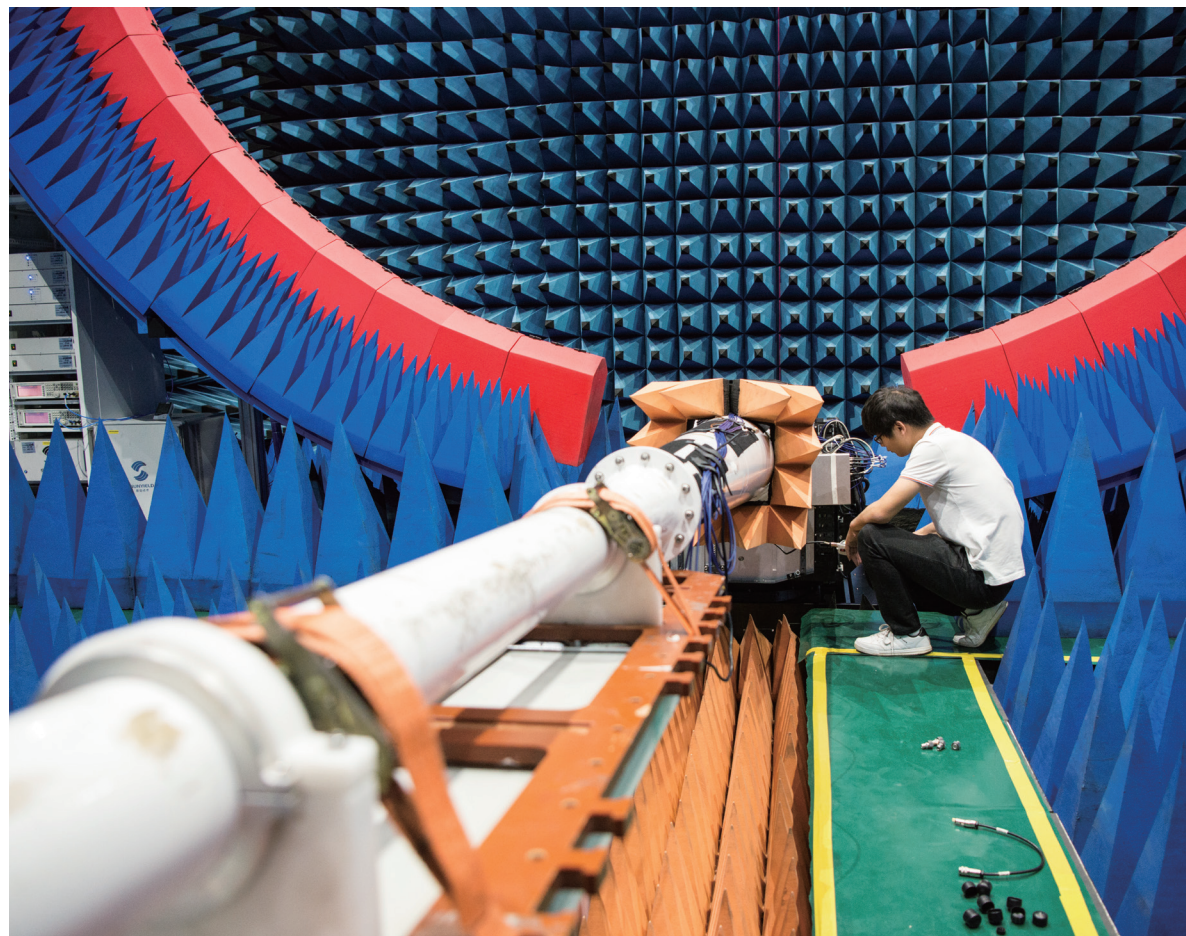
产业逐步迈向高质量发展。图为通宇通讯公司工作人员正在检测天线。(图/周宏尚)
